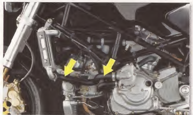
Mangueras
